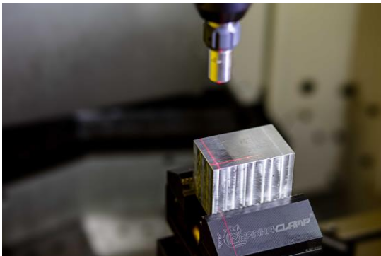
Das Laserkreuz des Lasertasters ermöglicht einfaches, schnelles und kontaktloses Antasten.
