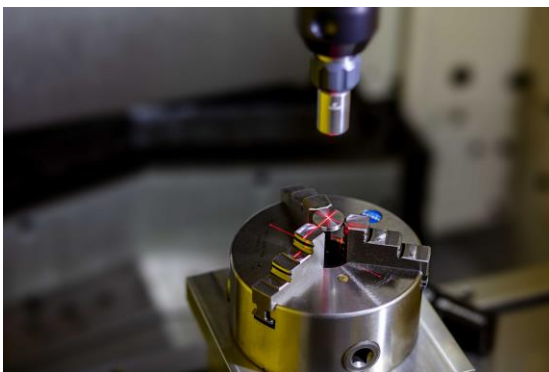
Auch zur Bestimmung des ungefähren Mittelpunktes eines runden Werkstückes eignet sich der Tschorn Lasertaster.
